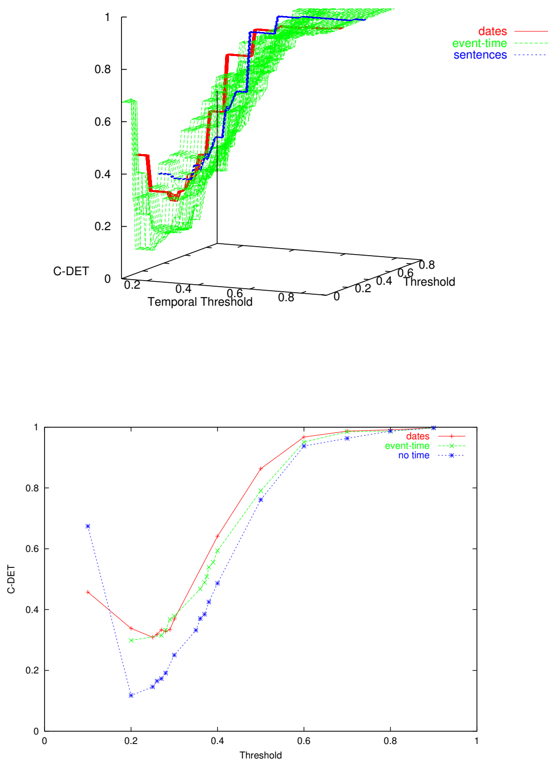
Figura 5.14: Coste de detección de tópicos.
