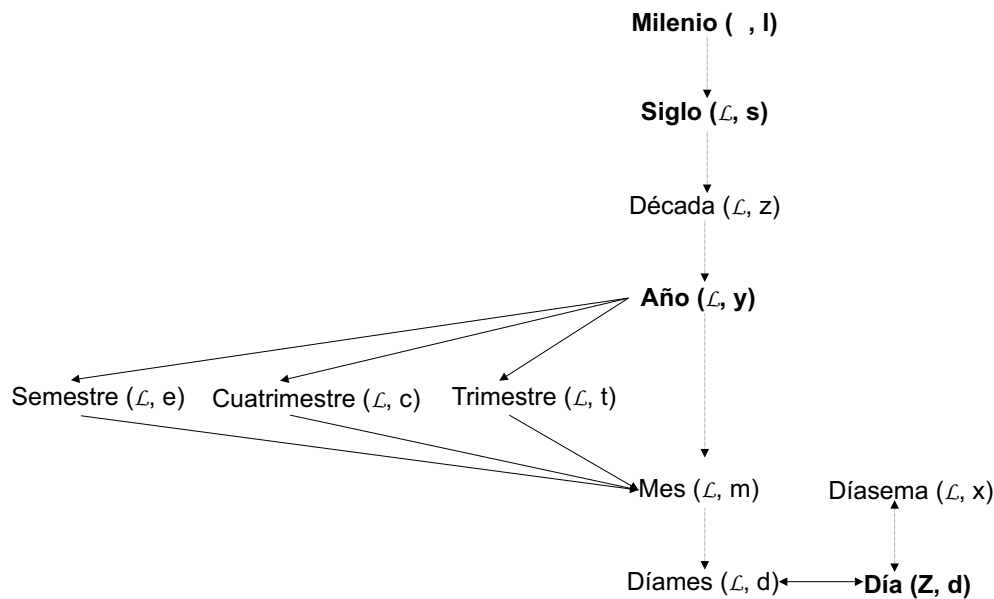
Figura 3.1: Grafo dirigido por la relación \bar{\wedge} entre las granularidades del calendario Gregoriano.
